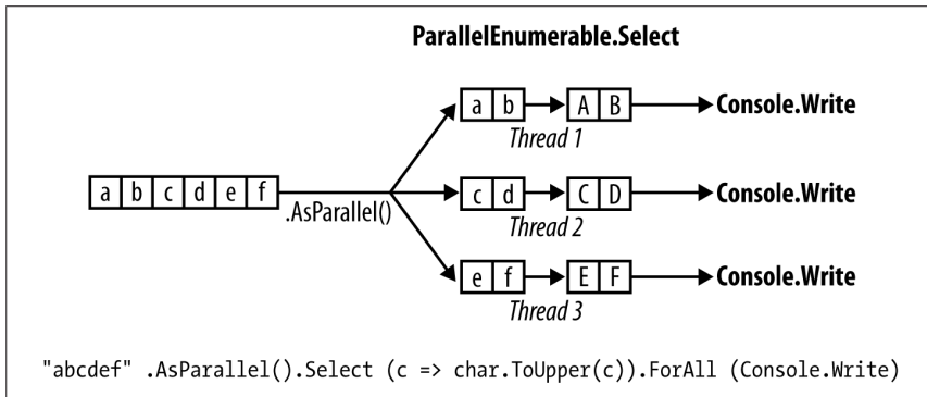
Figure 23-3. PLINQ ForAll
